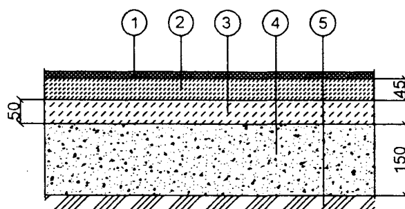
Схема 2. Пол по перекрытию
