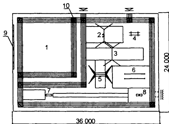
ЗАЛ 24×36 м ДЛЯ СПОРТИВНОЙ ГИМНАСТИКИ
