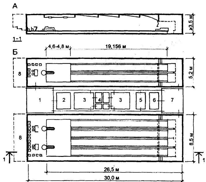
Планировочная схема кегельбана
