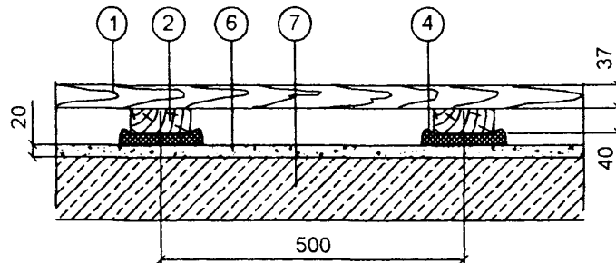
Схема 2. Пол по двойным лагам
