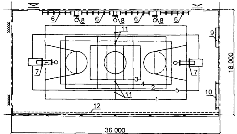
СХЕМА РЕШЕНИЙ ЗАЛОВ ДЛЯ ОФП И ТРЕНИРОВОК
