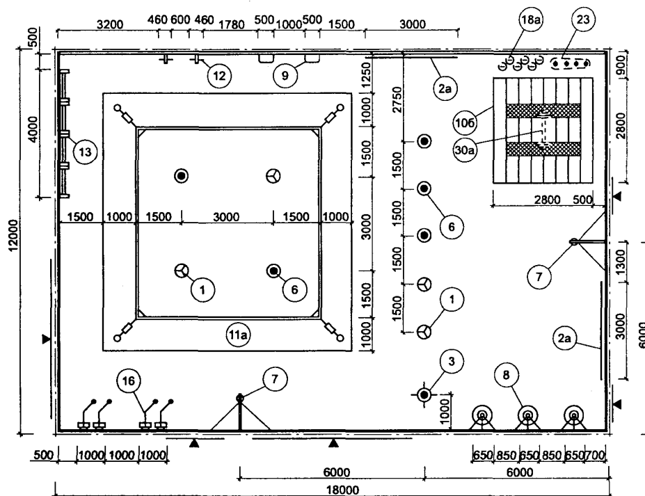
ПЛАН ЗАЛА 18×12 м ДЛЯ УЧЕБНО-ТРЕНИРОВОЧНЫХ ЗАНЯТИЙ
