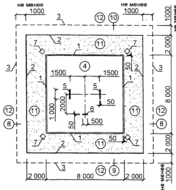
СХЕМА ПЛАНА АРЕНЫ ДЛЯ СОРЕВНОВАНИЙ ПО ДЗЮДО
