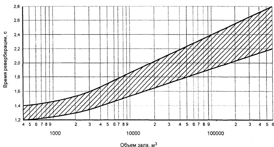
Рисунок 7.1 — График времени реверберации
