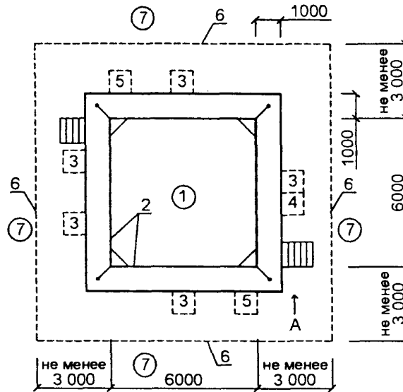
СХЕМА ПЛАНА АРЕНЫ ДЛЯ СОРЕВНОВАНИЙ ПО БОКСУ
