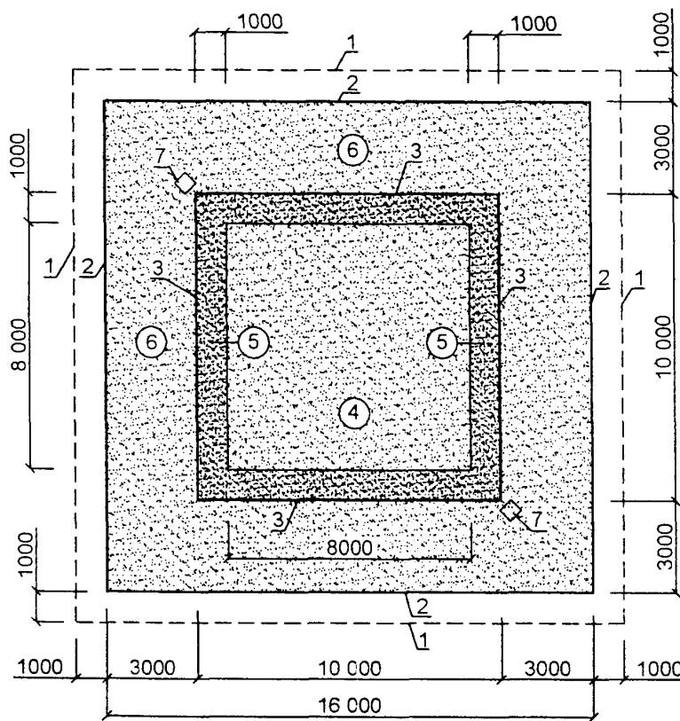
СХЕМА ПЛАНА АРЕНЫ ДЛЯ СОРЕВНОВАНИЙ ПО ДЗЮДО
