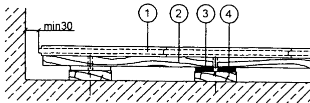
Схема 3. Пол на амортизирующей подложке
