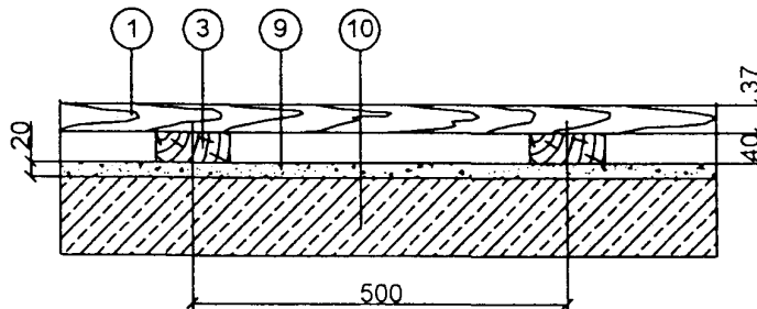
Схема 3. Брусчатый пол по лагам на грунте
