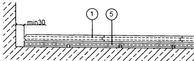
Схема 3. Пол на амортизирующей подложке
