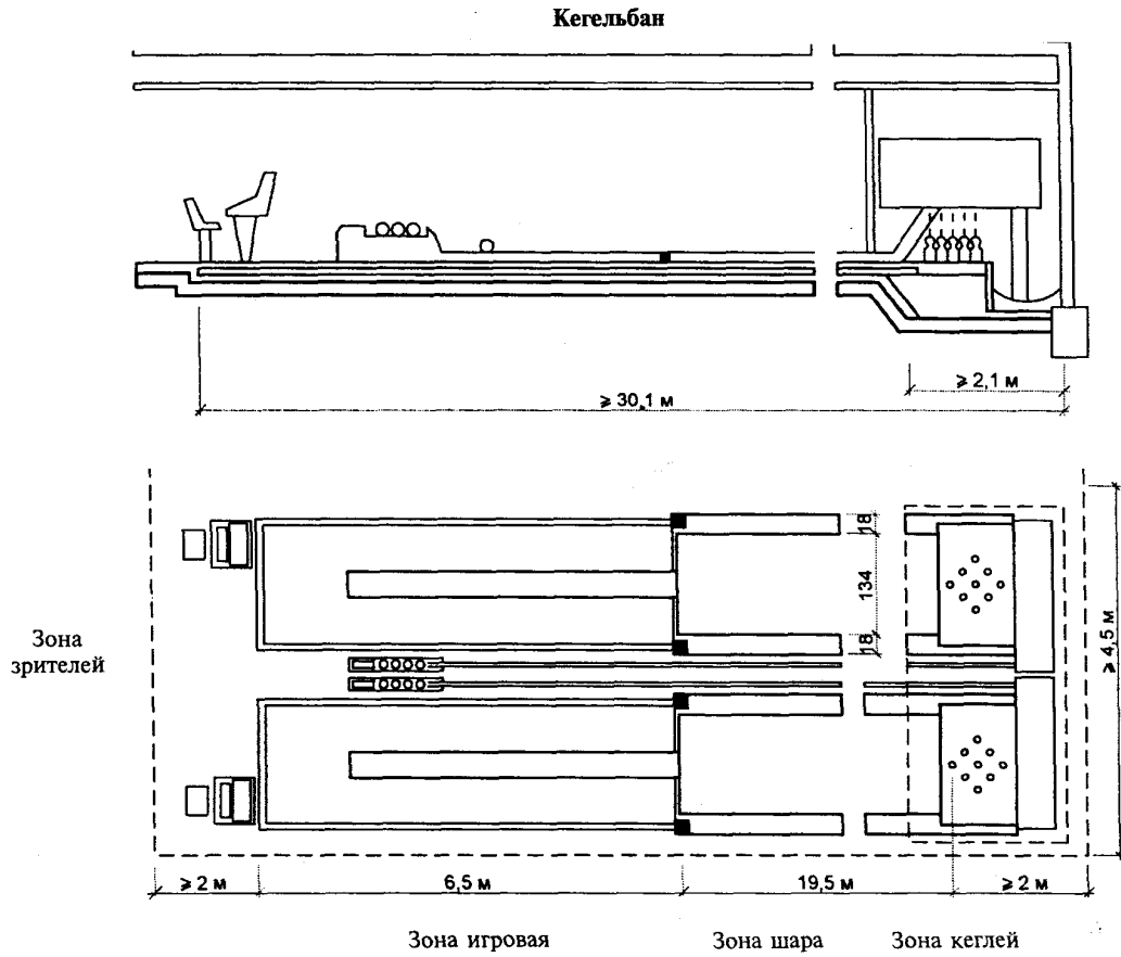
Планировочная схема кегельбана
