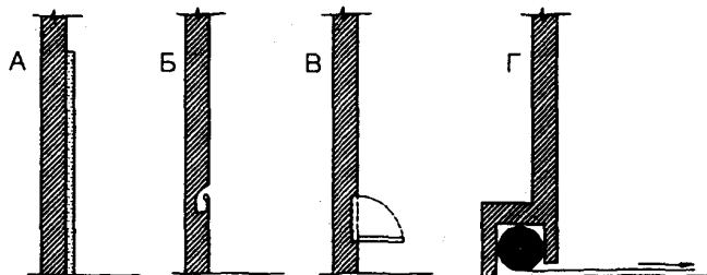
Особенности решения стен спортивных залов
