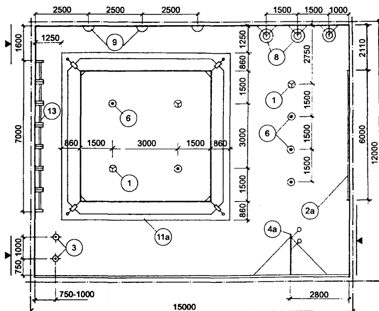
ПЛАН ЗАЛА 15×12 м ДЛЯ УЧЕБНО-ТРЕНИРОВОЧНЫХ ЗАНЯТИЙ
