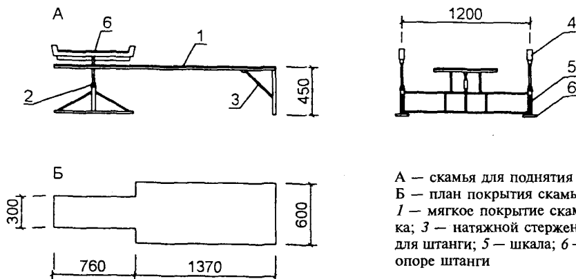
Скамья для занятий тяжелой атлетикой
